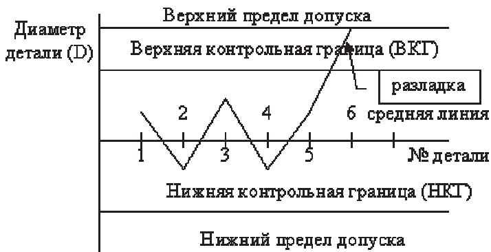
Рис. 4.20. Пример контрольной карты
