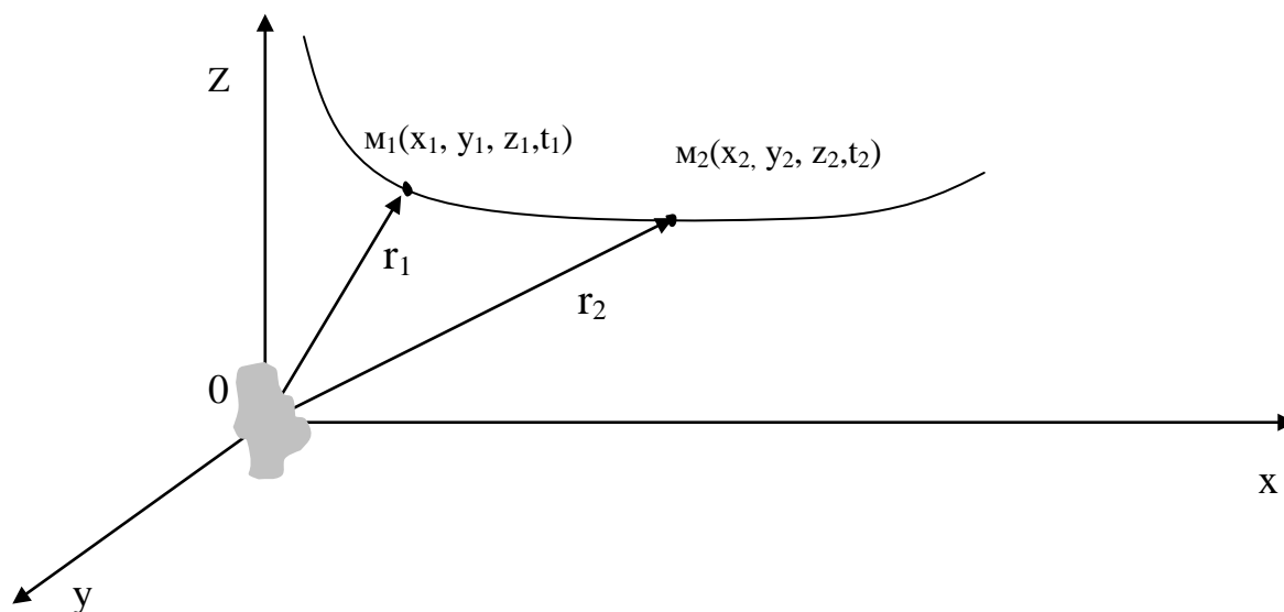
Рис. 1. Система отсчета
